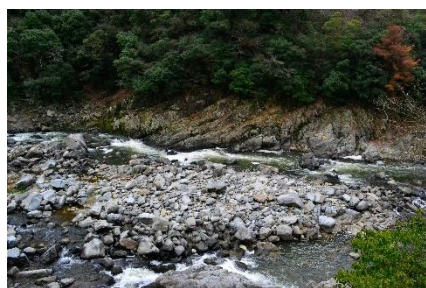
廃線跡案内板付近 溶結凝灰岩
