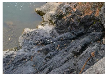
第8トンネル出口付近 泥岩 丹波層群 (約2億5000万年前)
